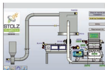
Supervisor WinCC (a petición)
